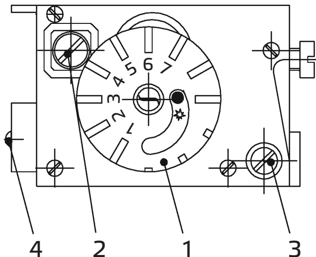
Рисунок 2 — Блок газовый
