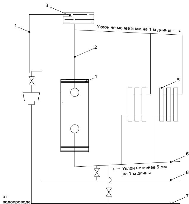
1 — сигнальная труба; 2 — главный стояк; 3 — расширительный бак; 4 — аппарат; 5 — радиатор; 6 — трубопровод обратной воды; 7 — сливная магистраль; 8 — водопровод подпиточный
