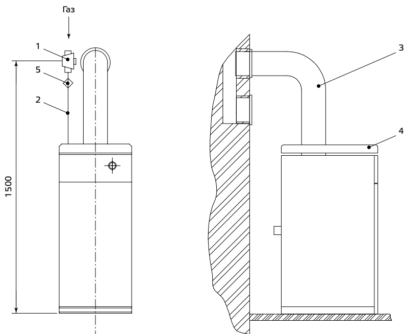
1 — газовый кран; 2 — газоотводящая труба; 3 — дымоотводящая труба; 4 — аппарат; 5 — фильтр газа
